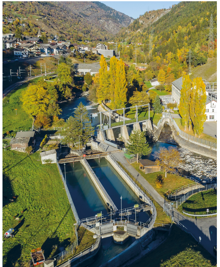
Dans le cadre du projet HydroLEAP, le remplacement de l'actuelle turbine Francis par une turbine Pelton est testé dans la centrale hydroélectrique au fil de l'eau à haute pression d'Ernen, dans le Haut-Valais. Il s'agit ainsi d'acquérir de l'expérience pour des mesures de réaménagement dans d'autres centrales hydroélectriques suisses. Photo: FMV
